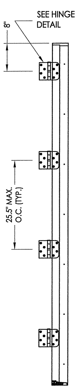
HINGE JAMB
